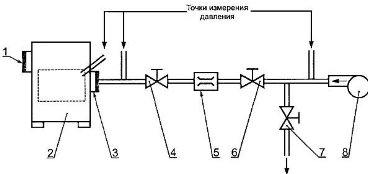
Рисунок 4 - Схема стенда для испытания котлов на газоплотность
