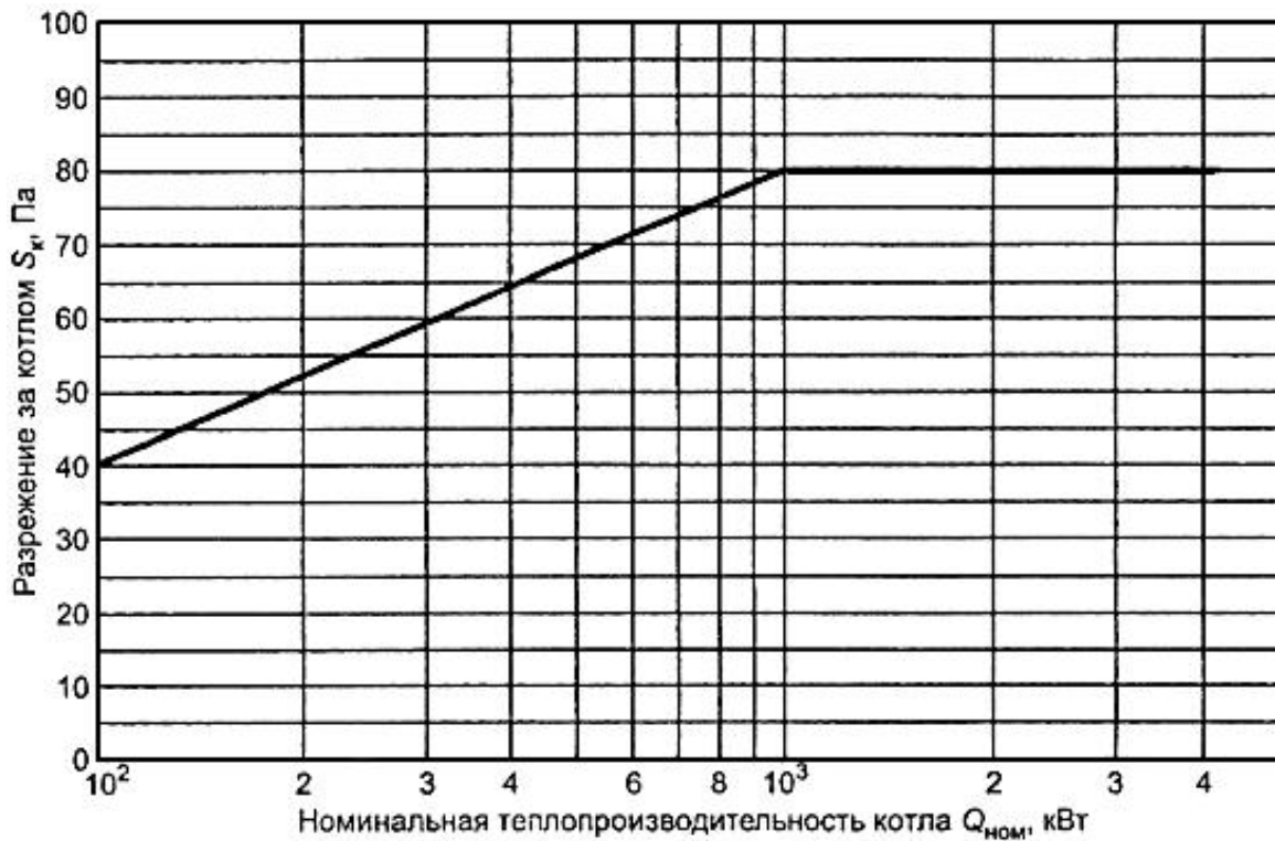
Рисунок 2 - Максимальное разрежение за котлом на естественной тяге
